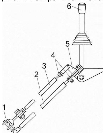
Рисунок 2.10 – Механизм переключения передач
